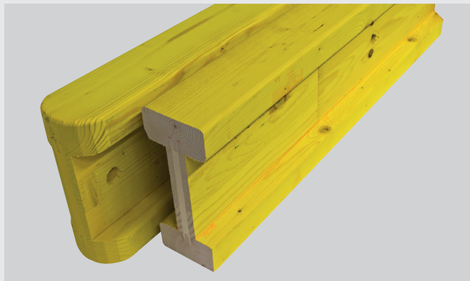
Traverse réalisée en panneaux de 3 couches, avec attaches talon à clavettes zinguées pour assurer une grande stabilité et une durabilité des poutrelles PF20 et H20 top.
